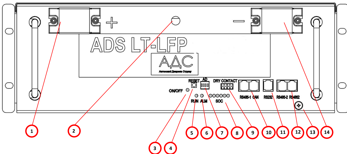
Рис.2-3 Зображення панелі управління
